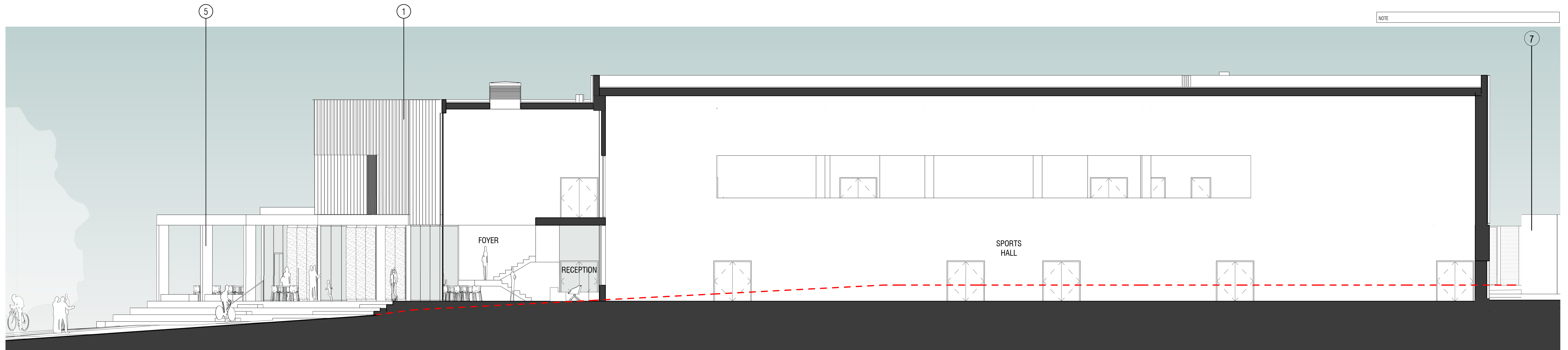
CC 1:100
